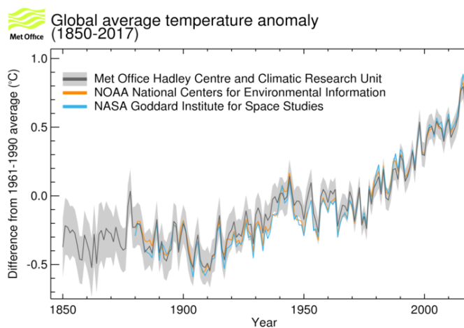
Rys. 1. Anomalia średniej rocznej temperatury Ziemi w odniesieniu do średniej temperatury z okresu 1961–1990. Dane trzech z głównych ośrodków badawczych: Met Office, NOAA i NASA. Źródło ilustracji: Met Office.
