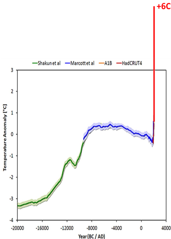
Rys. 3. Zmiany temperatury w ostatnich 22 000 latach. Źródła: Shakun 2012 (linia zielona), Marcott 2013 (linia niebieska), HadCRUT4, przedłużenie w przyszłość w oparciu o scenariusz RCP8.5 Meinshausen 2011 (linia czerwona). Źródło: portal Nauka o Klimacie: http://naukaoklimacie.pl .
