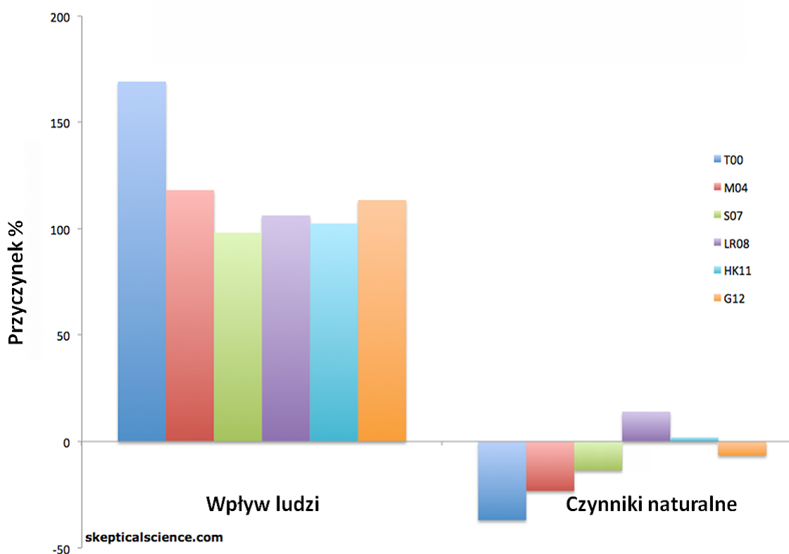
Rys. 2. Przyczynki antropogeniczne i naturalnych procesów do obserwowanego ocieplenia powierzchni Ziemi w ciągu ostatnich 50–65 lat, według: Tett i in. 2000 (T00, ciemny niebieski), Meehl i in. 2004 (M04, czerwony), Stone i in. 2007 (S07, zielony). Źródło: portal Nauka o Klimacie: http://naukaoklimacie.pl .
